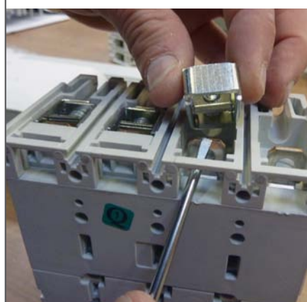
Retirer les bornes à cages amont.
