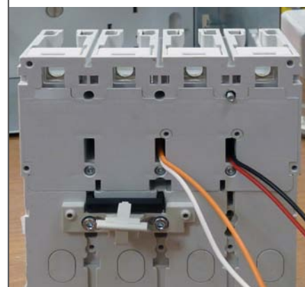
Retirer des bornes à cage amont et aval.
