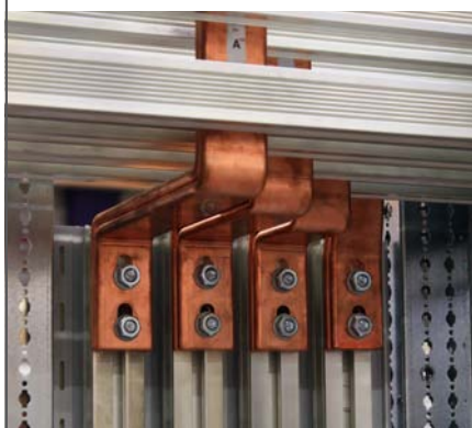
Montage du kit de raccordement réf. 4 046 93. Couples de serrage : 50 N · m
