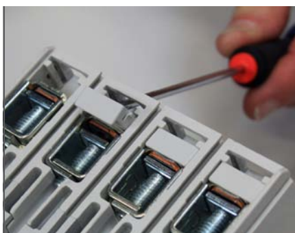
Retirer les obturateurs arrière amont et aval.
