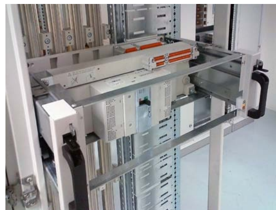
BASE IS 333 EN POSITION "DÉBROCHÉ"
