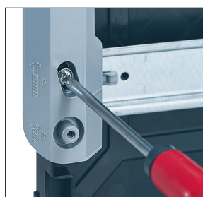
2 CHASSIS AMOVÍVEL Permite a instalação e cablagem dos dispositivos em oficina. Ajuste da posição graças aos orifícios oblongos.
