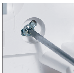
3 AJUSTE DE POSIÇÃO E MODELO DE INSTALAÇÃO Ajuste de posição graças aos orifícios oblongos. Medidas dos eixos de fixação marcados no fundo do quadro.
