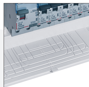
6 PASSAGEM DAS CALHAS Entradas com pré-cortes para passagem das calhas por baixo ou por cima, dependendo da posição do quadro.
