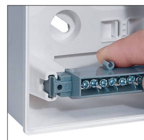
4 LIGADORES HORIZONTAIS Quadros equipados com ligadores terra e neutro. Instalação fácil sem ferramentas.
